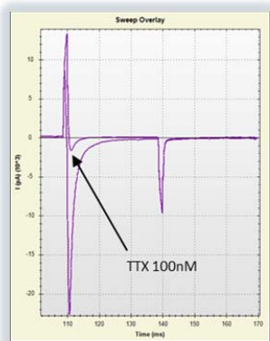
Figura 23. Efecto de la TTX sobre los canales Nav a estudio. A) Registros de corriente solapados de los barridos con solución externa inmediatamente antes de añadir la TTX. B) Gráfica de incremento de corrientes del canal abierto (pico) menos canal cerrado (basal) en el curso del experimento. El cursor azul en el compuesto 7 (C7), marca el momento de adición de TTX 100 nM, reflejado en la gráfica A en el pico casi nulo. En el compuesto 2 (C2), se aprecia la presencia de un bloqueador suave.
