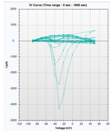
Figura 29. Registros y curva IV de CHONa1.6wt. A) Registros de la corriente de sodio a distintos voltajes sin ajustar a línea basal. B) Curva IV obtenida del software con el pico máximo de corriente a - 30 mV.
